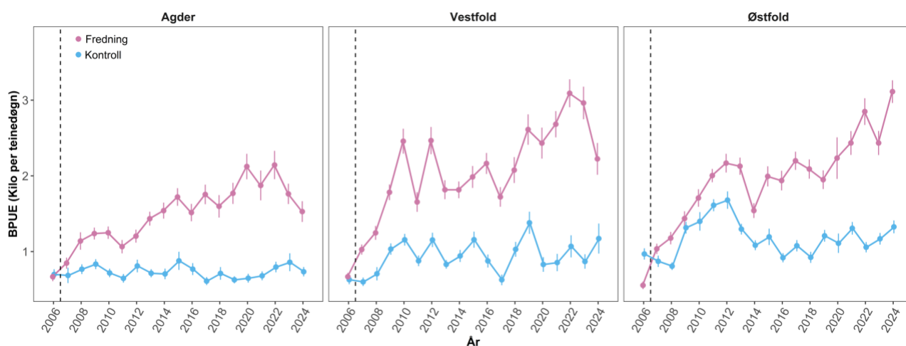
Figur 19: Biomasse (kg) av hummer per teine i Flødevigen (Agder), Bolærne (Vestfold) og Kverniskjær (Østfold) i fredningsområder og kontrollområder i perioden 2006 til 2024. Loddrett stiplet linje indikerer etablering av hummerfredningsområder (2006). Oppdatert av Sørvalen fra Knutsen et al. (2022).
