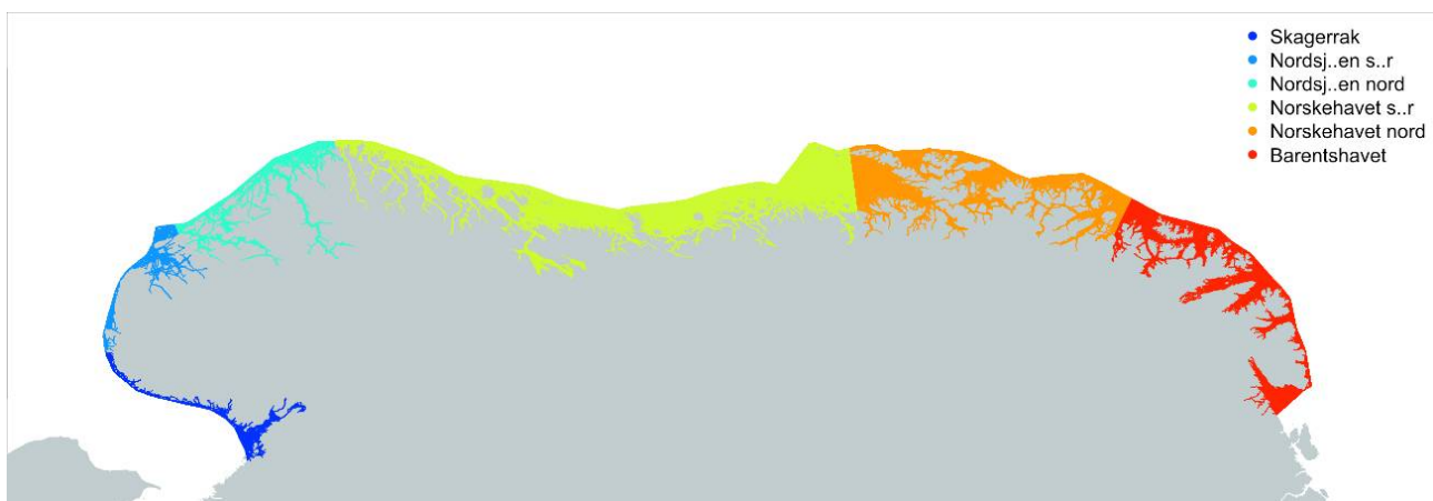
Figur 3 . Økoregioner bestemt for kystvann i Norge.
