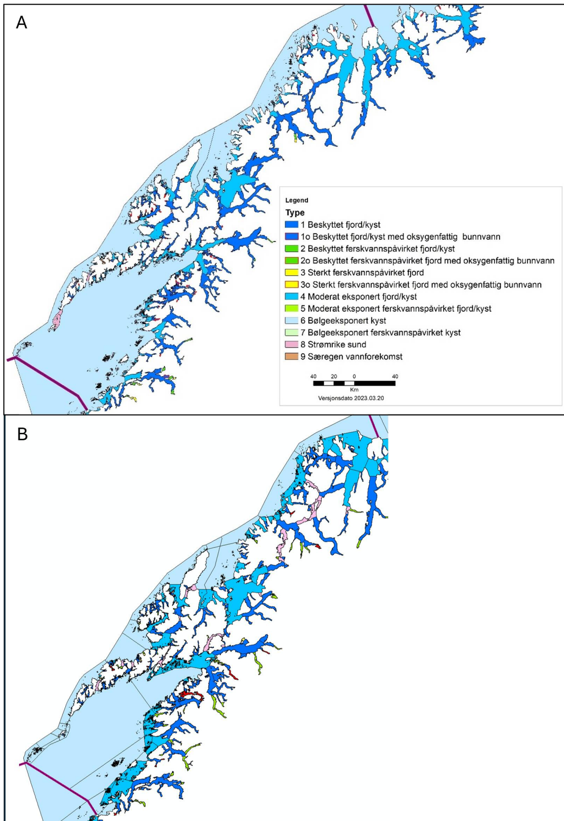
Figur 33. A) Kart over foreslåtte vann typer i region Norskehavet Nord (G) basert på modellerte faktorer. Til sammenlikning B) dagens vann typeinndeling (2019). Ikke alle vann typer eksisterer i alle regioner.
