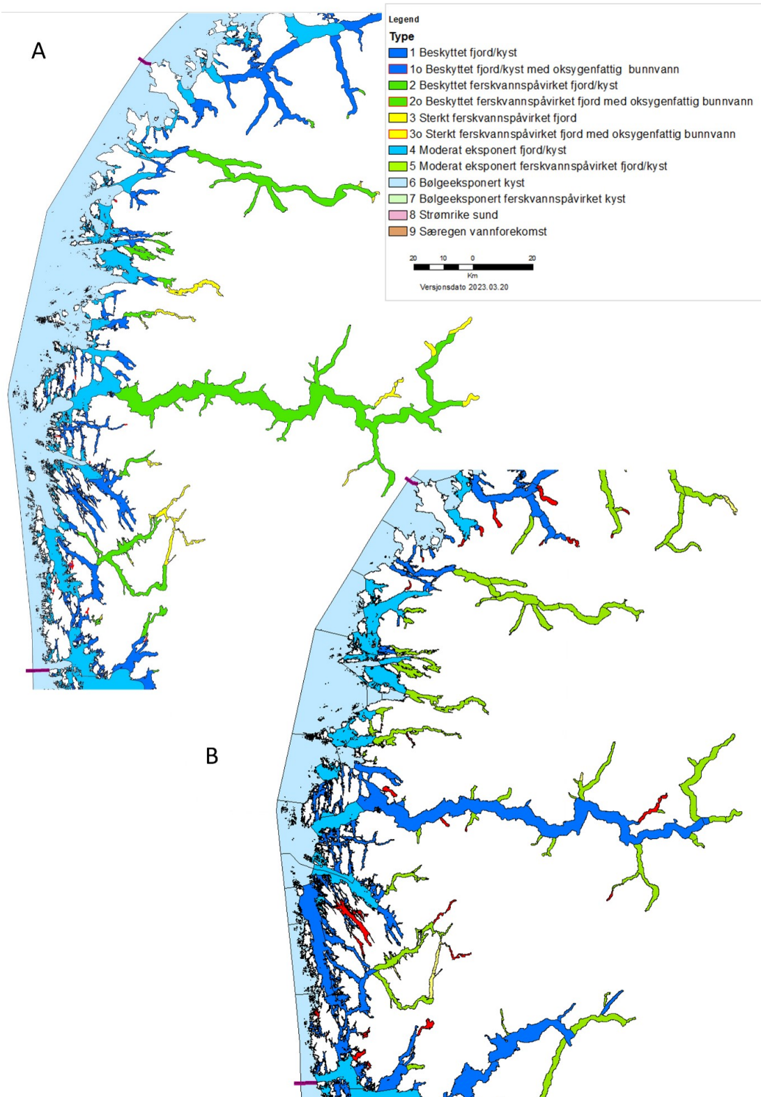
Figur 35. A) Kart over foreslåtte vanntyper i region Nordsjøen Nord (M) basert på modellerte faktorer. Til sammenlikning B) dagens vanntypeinndeling (2019). Ikke alle vanntyper eksisterer i alle regioner.
