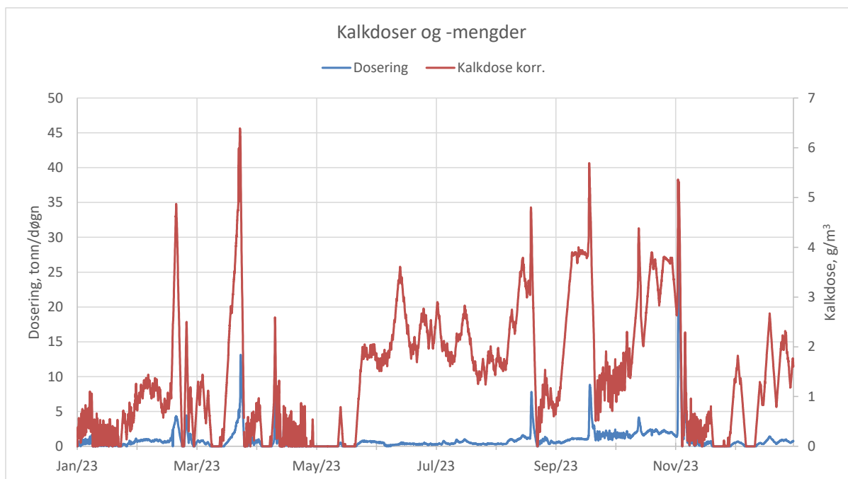
Figur 7. Kalkdosen fra anlegget ( \text{g/m}^3 ) vist sammen med total mengde utdosert kalk per døgn (tonn).
