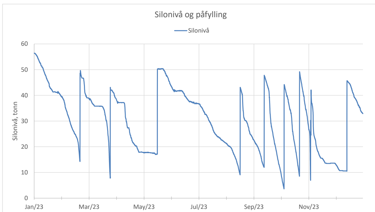
Figur 8. Oversikt over silonivå og påfyllinger i løpet av året.
