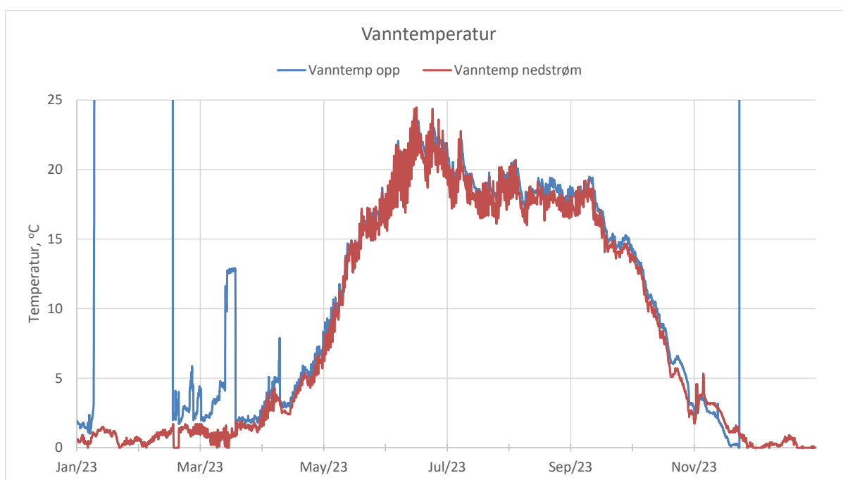
Figur 2. Vanntemperatur oppstrøms Hauglandsfoss doseringsanlegg og nedstrøms ved Monane i 2023. Vertikale linjer skyldes forstyrrelser eller feil på signalet fra temperaturelementet.
