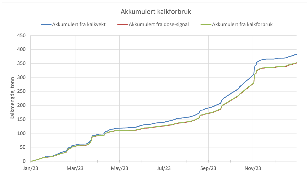
Figur 9. Akkumulert kalkforbruk beregnet på tre alternative måter: Fra (a) reduksjon av vekt i kalksilo, (b) dose-signal/styringsdose og (c) registrert kalkforbruk i tonn per/døgn.
