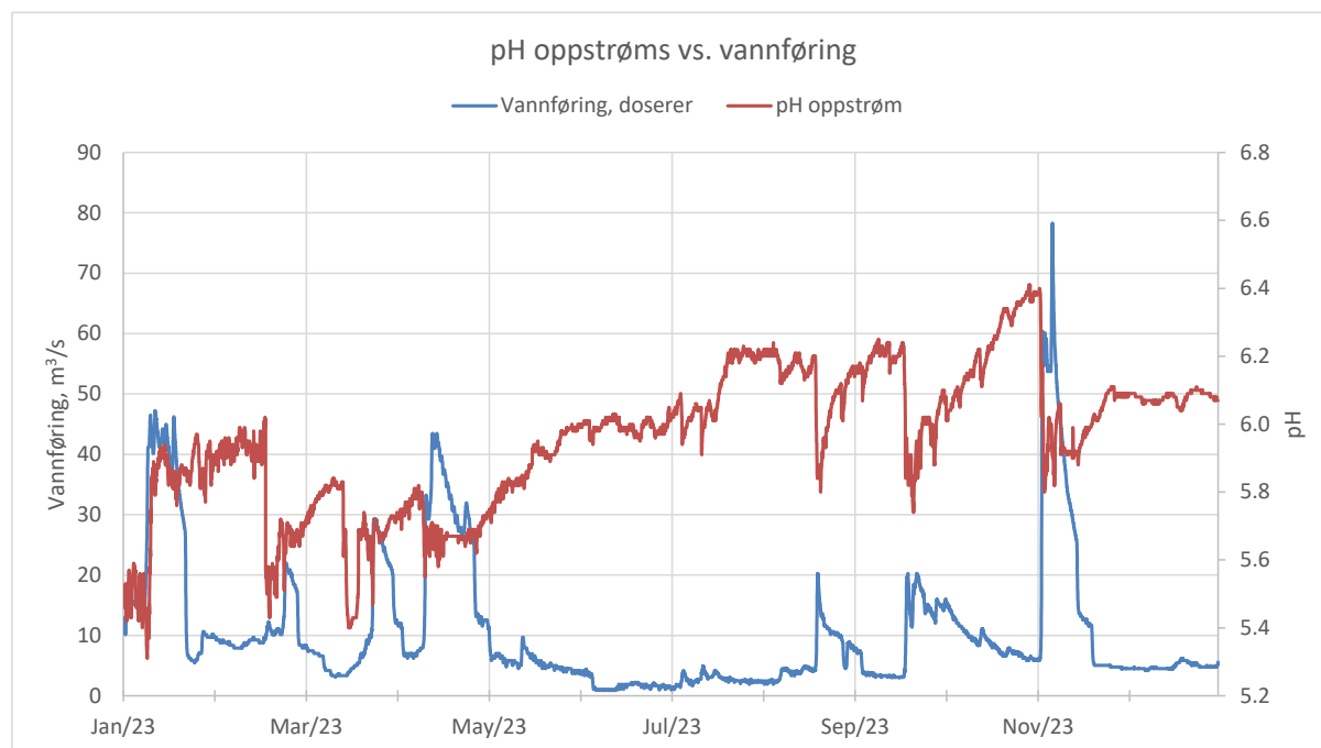
Figur 4. pH oppstrøms doseringsanlegget plottet sammen med vannføringssignalet til anlegget.
