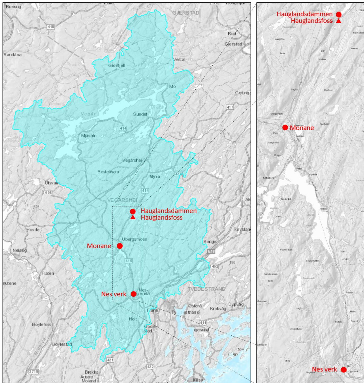
Figur 1. Vegårsfossdragnet nedbørfelt markert i blått, med plasseringer av kalkdoseringsanlegg (trekant) og pH-målestasjoner (sirkler). Kilde: https://temakart.nve.no/tema/nedbørfelt
