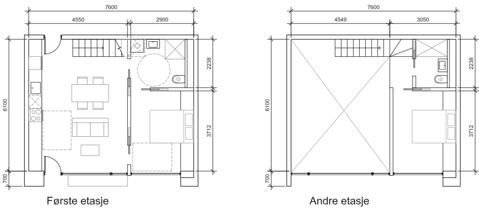
Planløsning for en typisk boligkjerne
