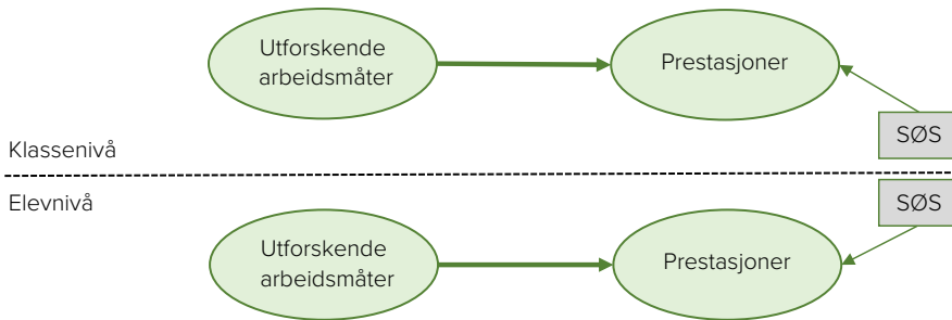
Figur 3.2 En analytisk modell om relasjoner mellom utforskende arbeidsmåter og elevers prestasjoner i naturfag på elev- og klassenivå, korrigert for SØS på begge nivåene.
