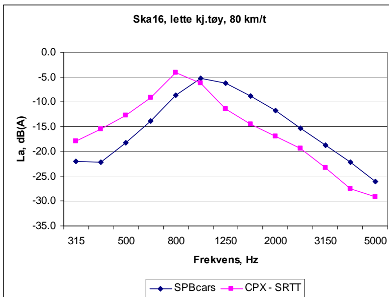
Figur 63 Veidekke73, Ska16. Normaliserte frekvensspektra for SPB_{lette} og CPX-SRTT. Lette kjøretøy ved 80 km/t
