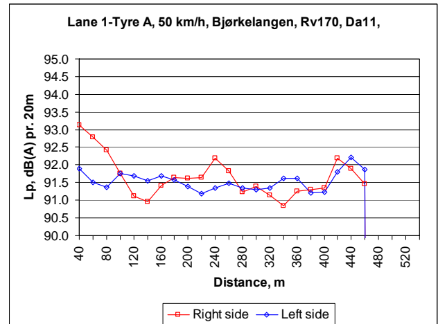
Figur 36 Veidekket 24, Da11, Alder: 1 år (2007)
