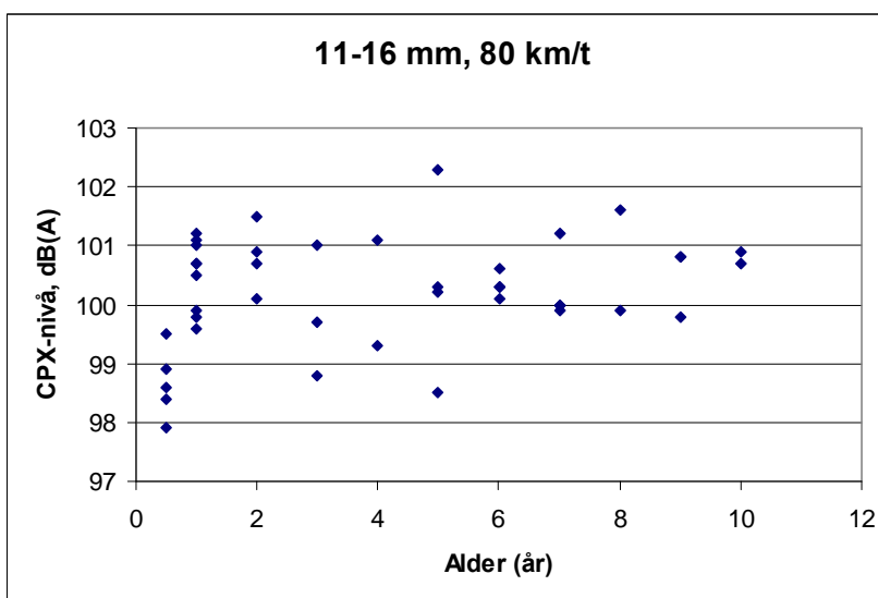
Figur 23 CPX-nivå for Ska/Ab-dekker 11-16 mm som funksjon av alder Hastighet: 80 km/t
