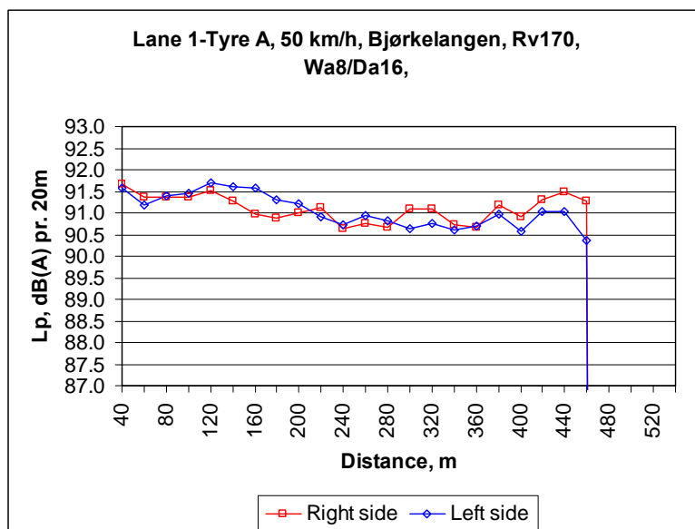
Figur 31 Dekke nr. 25: Wa8/Da16, Hastighet: 50 km/t. Måling i 2008 (to år gammelt)
