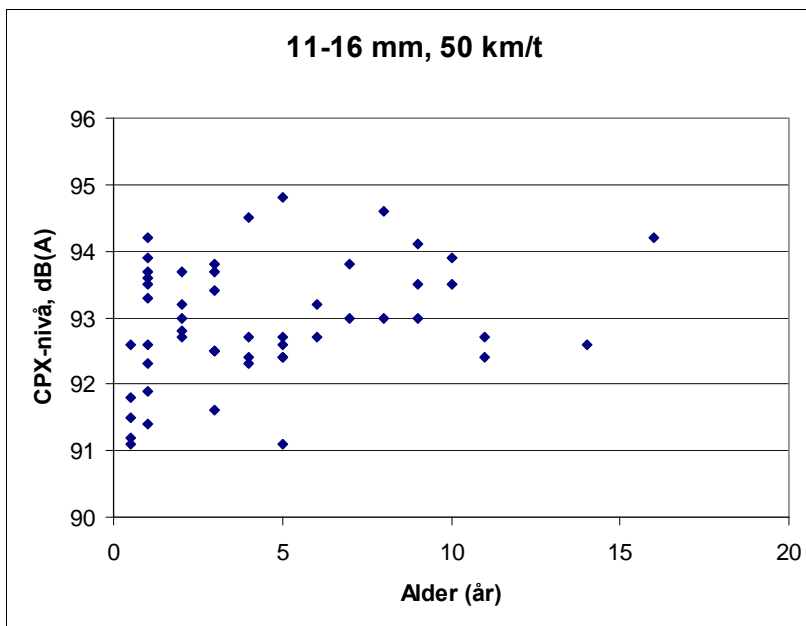
Figur 22 CPX-nivå for Ska/Ab-dekker 11-16 mm som funksjon av alder Hastighet: 50 km/t
