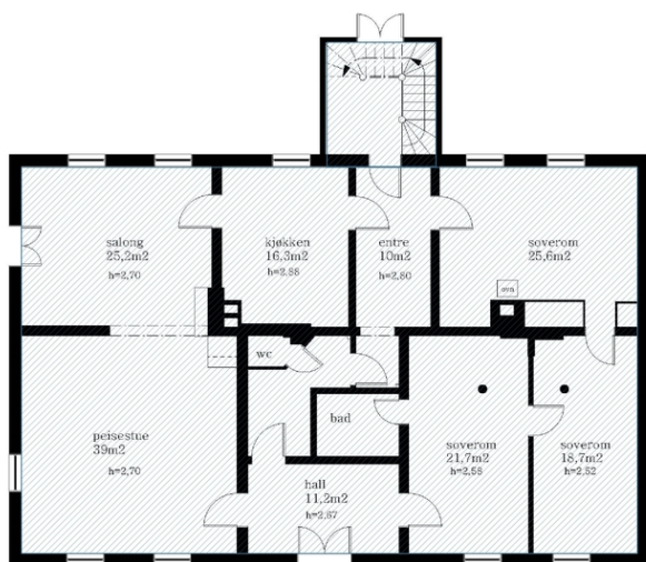
Plantegning med dagens situasjon (2009). 1. etasje. Opphavsrett: Statsbygg.
