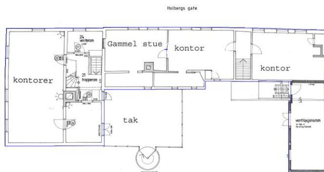
Plan andre etasje. Opphavsrett: Statsbygg.
