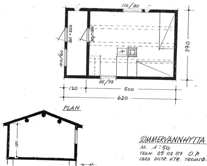
Plan- og snittegning. Opphavsrett: Reinpolitiet.
