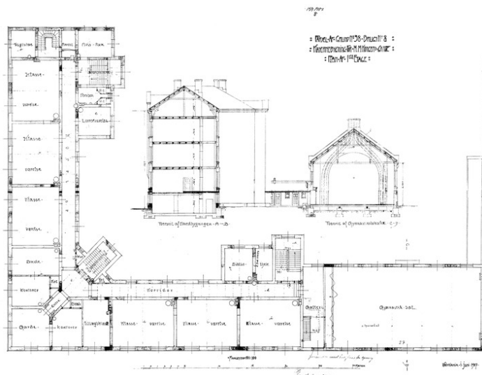
Plantegning for kasernen med gymnastikkbygning, 1. etg. Opphavsrett: Statsbygg.
