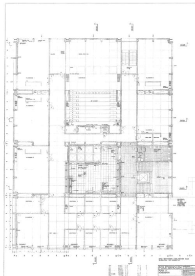
Plan 4. etasje. Opphavsrett: Statsbygg.
